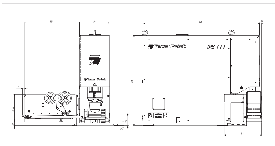
Das Bild auf der Vorderseite zeigt eine TPS 111 mit Tamponreinigung TAC. The picture on the front page shows a TPS 111 with pad cleaning device TAC.
